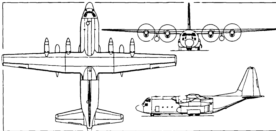
Figure II-3. Lockheed C-130E Hercules ( Jane's/Pilot Press ).
